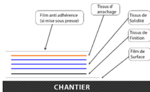
COUPE DE L'EMPLIAGE D'UNE PLAQUE STRATIFIEE
